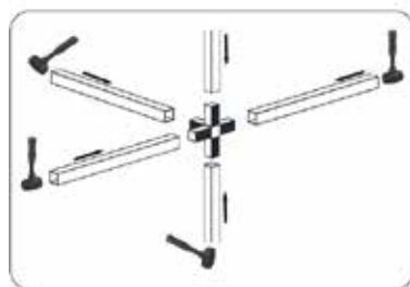
6 irányú csatlakozó
